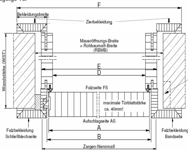
Einflügelige Tür
